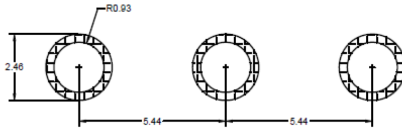
TO-247-3L
